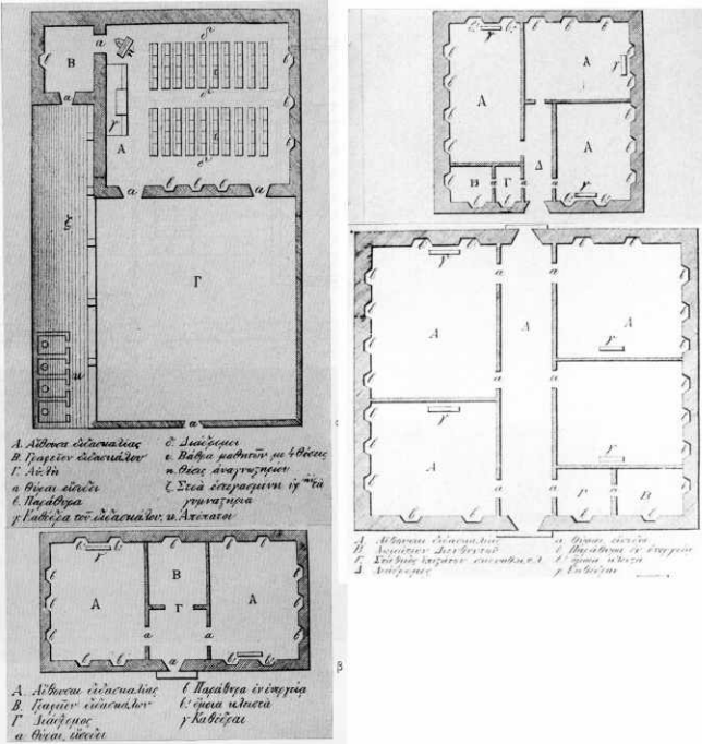
εικ. 2. Η οργάνωση του σχολικού κτηρίου σύμφωνα με τον Σπ. Μωραΐτη. α. Κάτοψη μονοτάξιου σχολείου β. Κάτοψη διτάξιου σχολείου γ. Κάτοψη τριτάξιου σχολείου δ. Κάτοψη τετρατάξιου σχολείου
