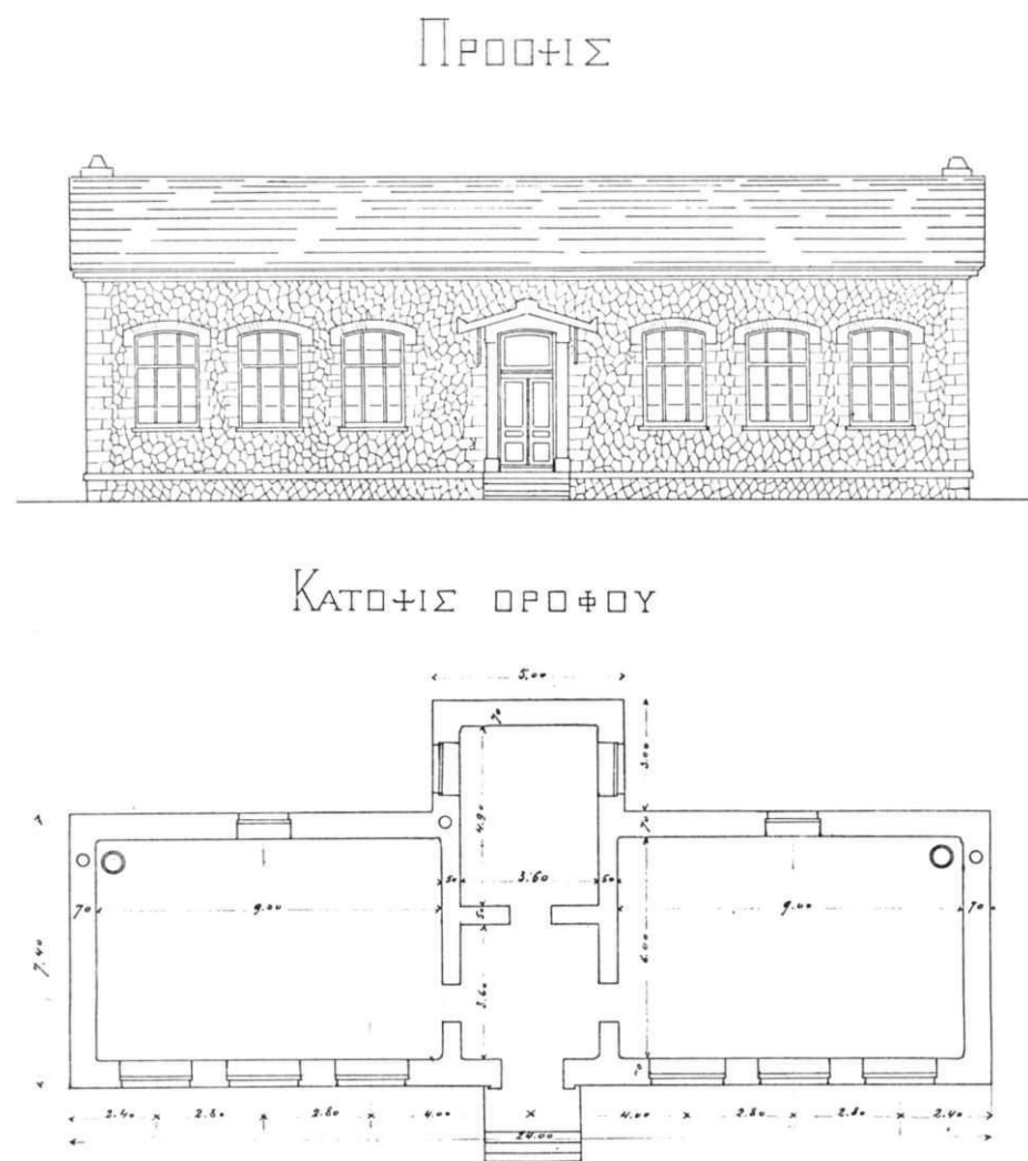
εικ. 5. Υπόδειγμα διτάξιου διδακτηρίου, 1911, (σειρά Α)
