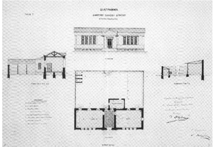
εικ. 3. α. «Τύπος Β'. Διάγραμμα σχολείου μονοτάξιου. Φωτισμός Μονοπλάγιος... Ο Νομομηχανικός Δ. Καλλίας. Εγκρίθηκε... 20 Απριλίου 1898». Λιθογραφία β. «Τύπος Γ'. Διάγραμμα σχολείου διτάξιου. Φωτισμός Μονοπλάγιος... Ο Νομομηχανικός Δ. Καλλίας... Εγκρίθηκε... 20 Απριλίου 1898». Λιθογραφία
