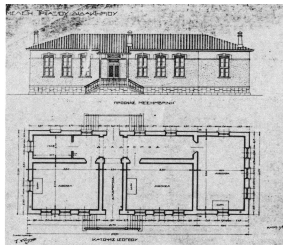
εικ. 6. Μελέτη τριτάξιου διδακτηρίου, τύπος 33. Αρχ. Π. Σούρσος, 1925
