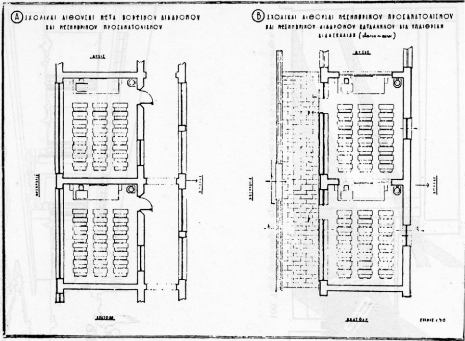
εικ. 6. Διάταξη και προσανατολισμός του διαδρόμου σε σχέση με τις αίθουσες: α. Τυπική διάταξη με αίθουσες μεσημβρινού προσανατολισμού και με κλειστό διάδρομο προς βορρά β. Διάταξη με ανοιχτό διάδρομο.
