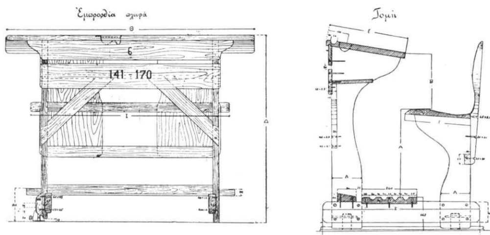
εικ. 4. Σχέδιο διέδρου θρανίου του Υπουργείου Δημοσίας Εκπαιδεύσεως, 1911
